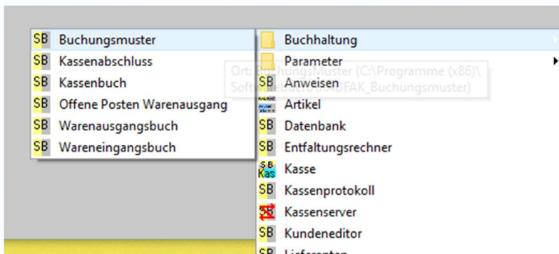
Abbildung 2 Oderstruktur Windows 7
