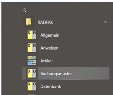
Abbildung 1 Startmenü Windows 10
